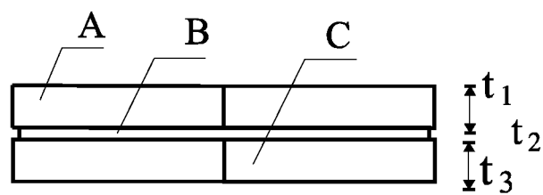
Poprečni presjek kroz panel
